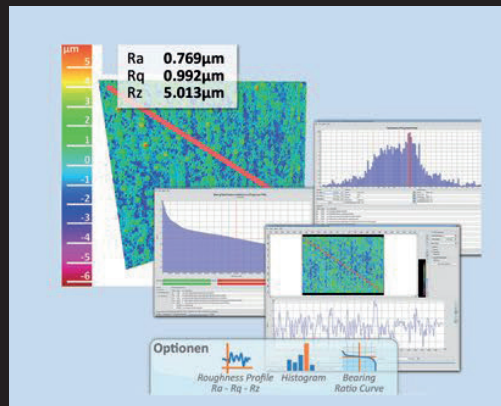
Linjska meritev hrapavosti
